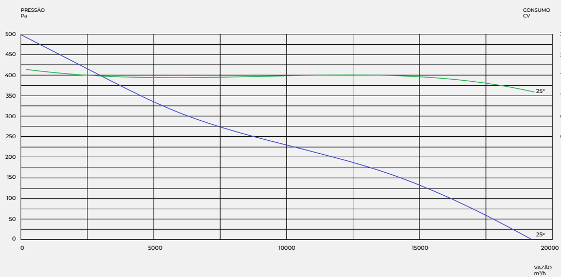
STG-AFS 800 AC/EC
