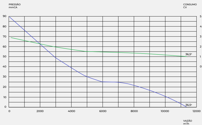
STG-AFSW 500 AC/EC
